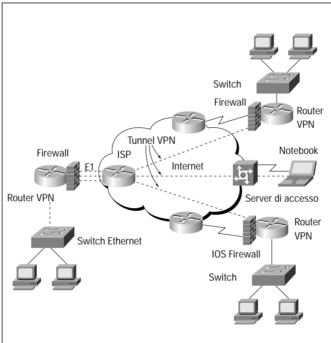
Figura 7: piccola VPN
